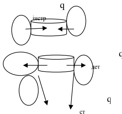
Рисунок 1 – Схема циркуляції теплових потоків, що виникають при різанні кераміки ВіМАО (вібромагнітнообразивна обробка): q_{\text{ст}} – тепло, що відводиться стружкою; q_{\text{дет}} – тепло, що поглинається деталлю; q_{\text{інстр}} – тепло, що поглинається інструментом
