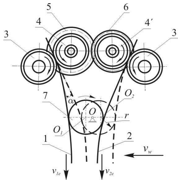
Рисунок 1 – Пристрій для наплавлення двома стрічковими електродами з контрольованим тепло- масоперенесенням електродного металу: 1, 2 – стрічкові електроди; 3, 3', 4, 4' – притиснічні роликки; 5, 6 – шестерні, 7 – ексцентриковий механізм
